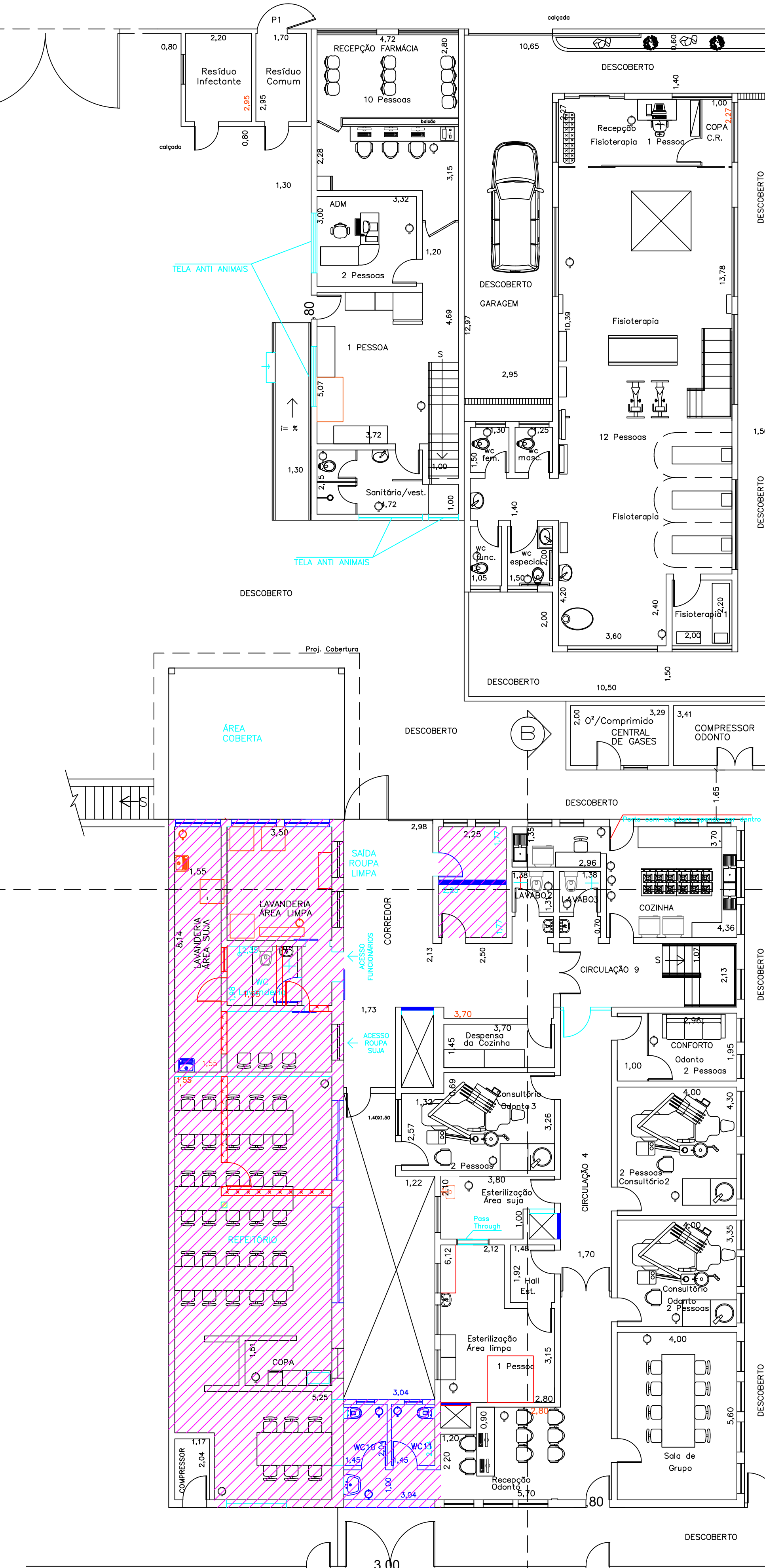
PAV. INFERIOR ESCALA 1/100
