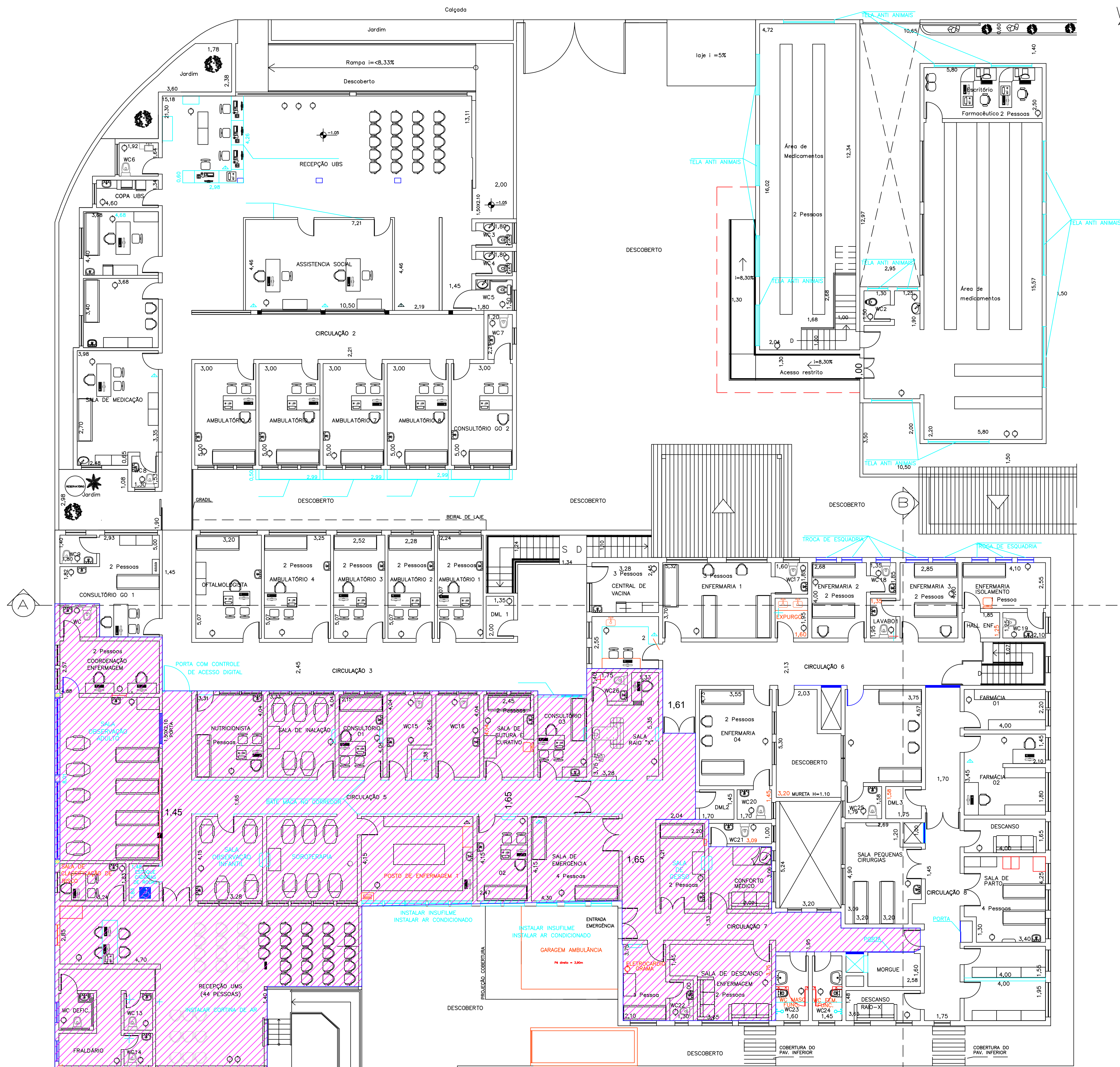
PAV. TÉRREO ESCALA 1/100
