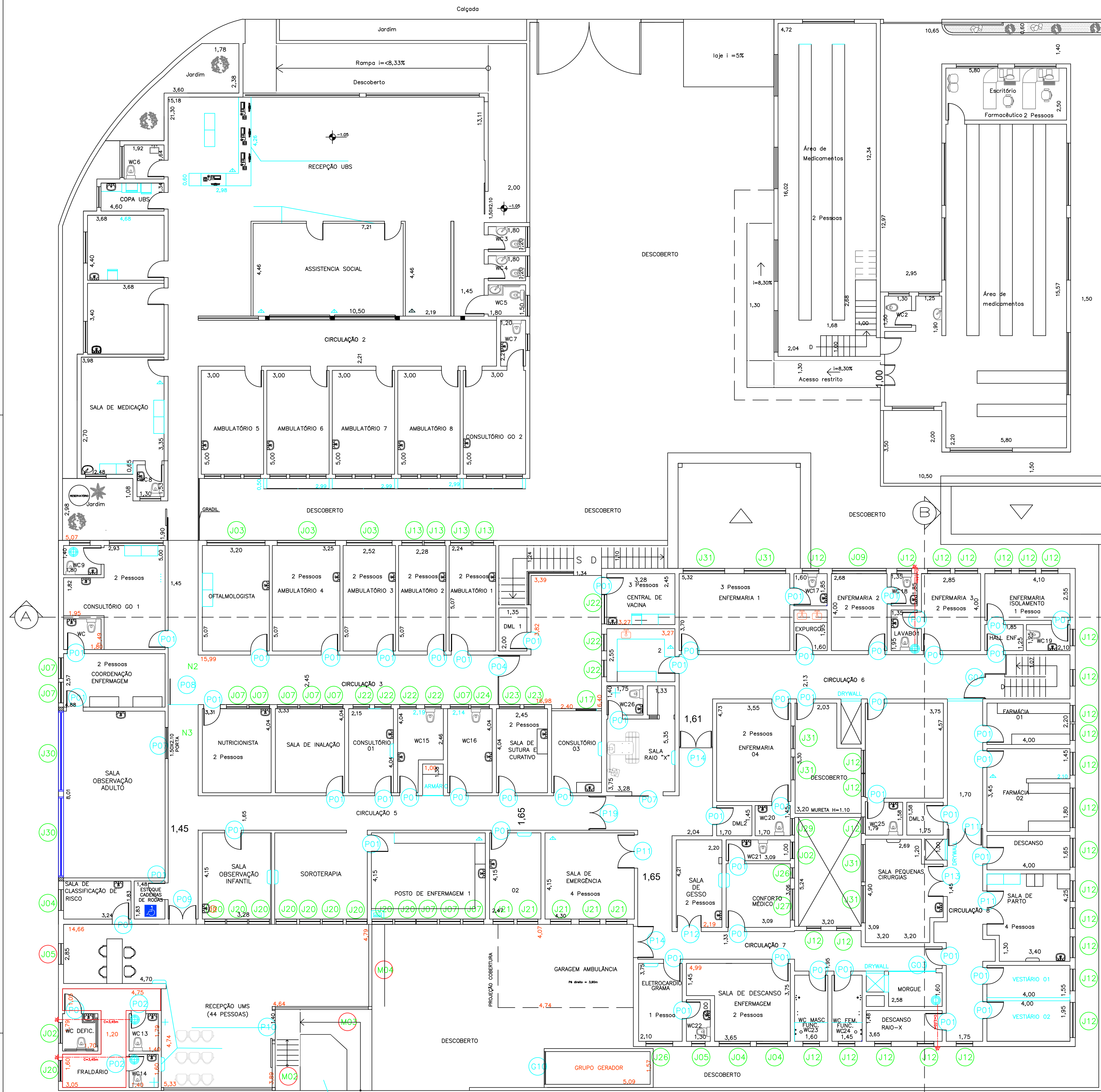
PAV. TÉRREO ESCALA 1/100
