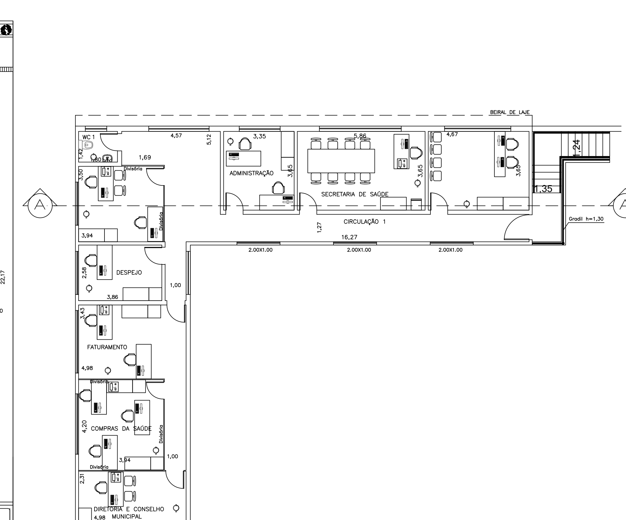
PAV. SUPERIOR ESCALA 1/100
