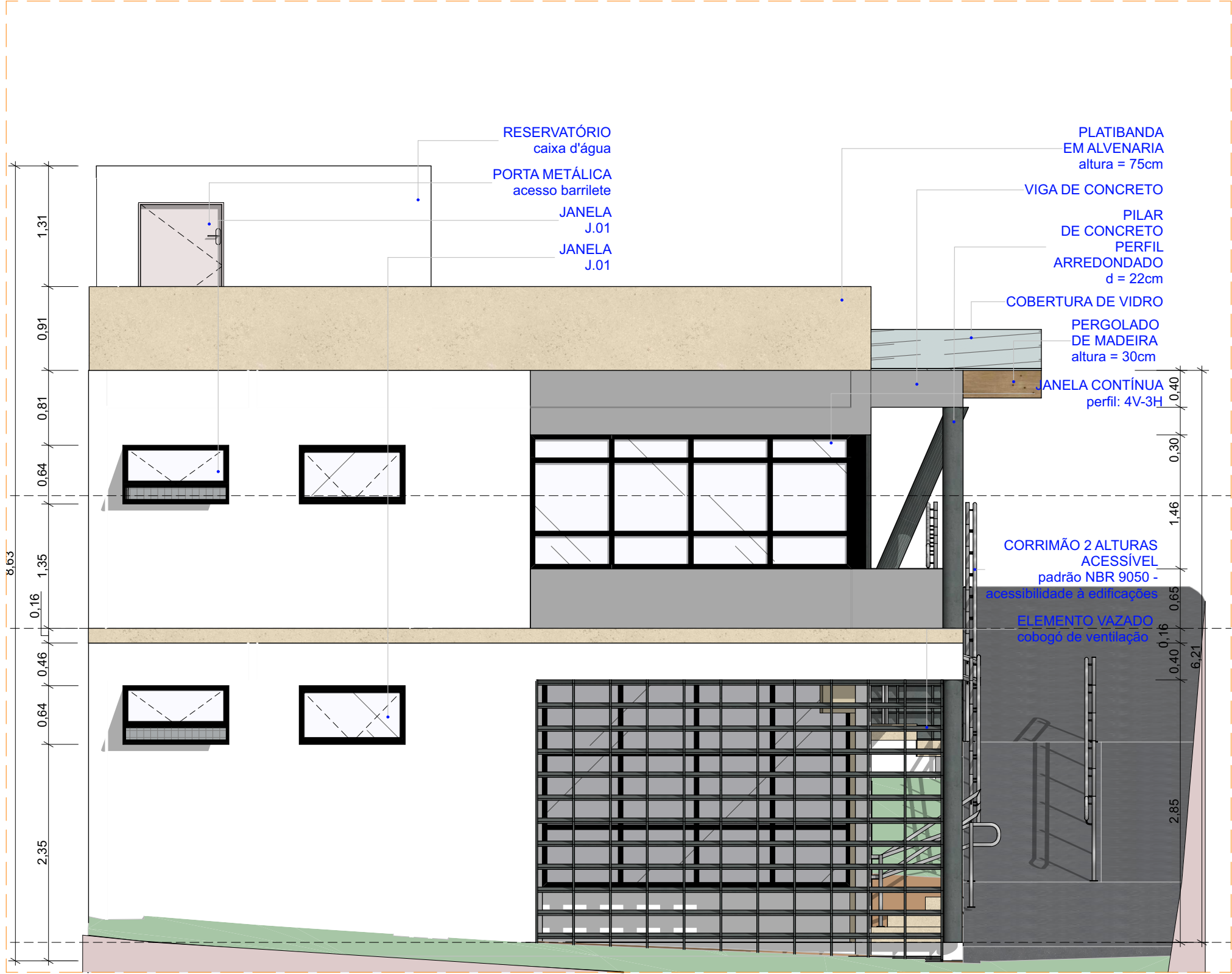
02 ELEVÇÃO - 04 Escala: 1:50
