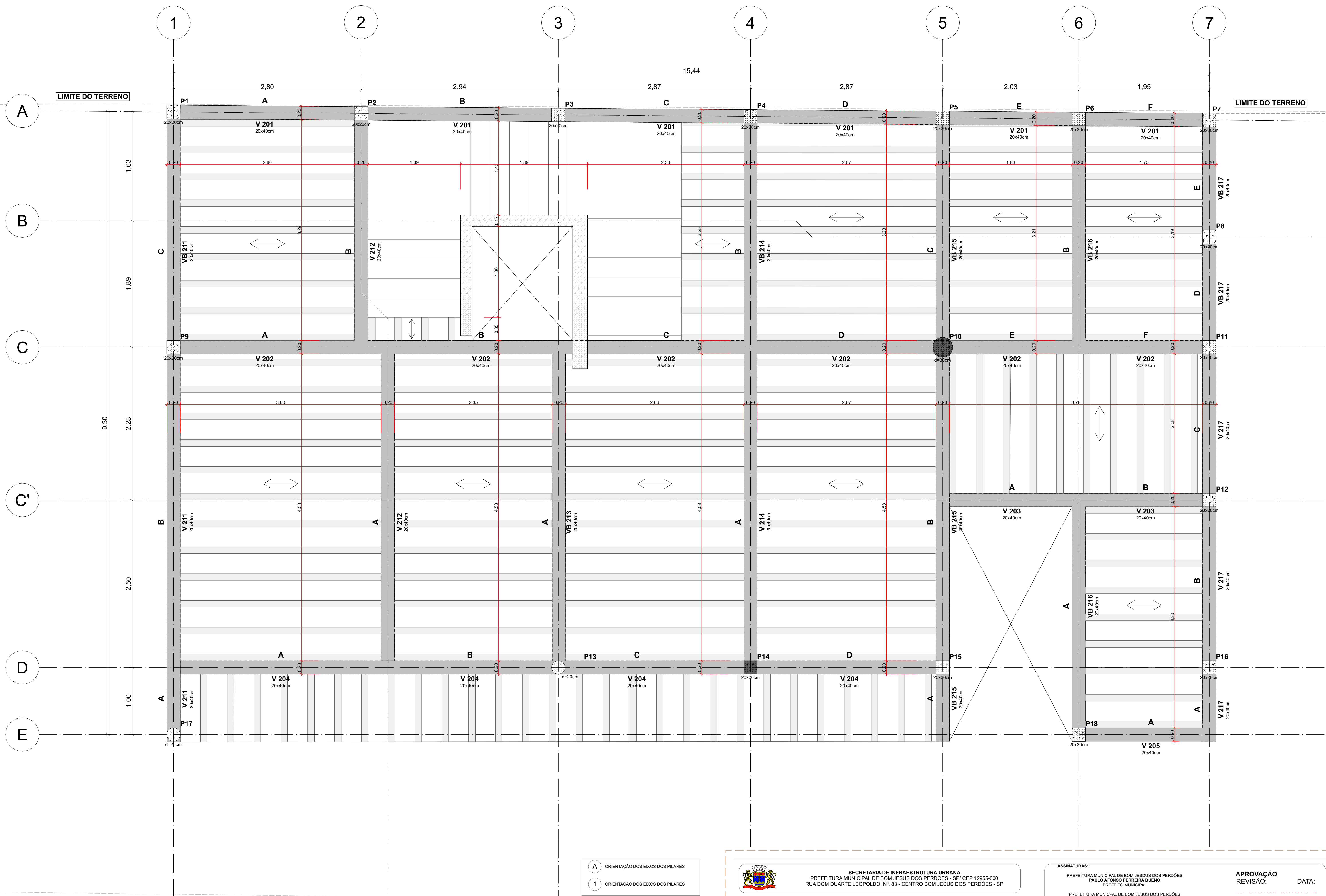
01 PLANTA DE FORMA PAV. SUPERIOR Escala: 1:25
