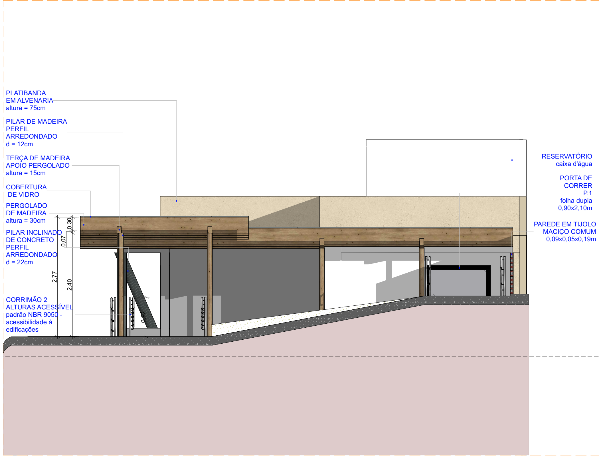
01 ELEVÇÃO - 02 Escala: 1:50
